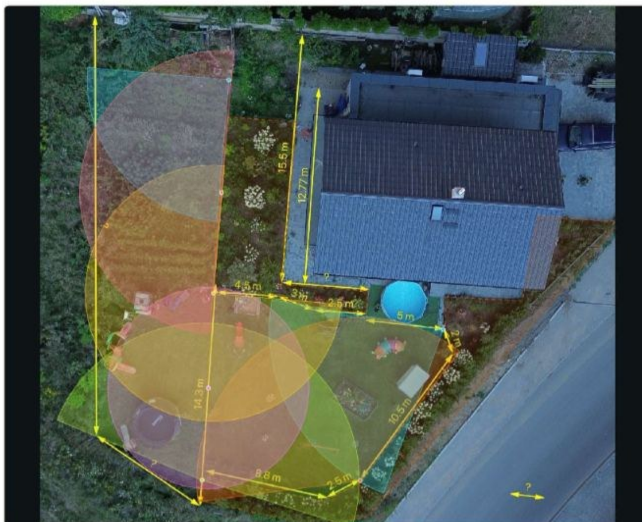
Rys. 1 — Projekt rozmieszczenia stref nawadniania na podkładzie z lotu ptaka. Kolorowe pola to zasięgi zraszaczy.
