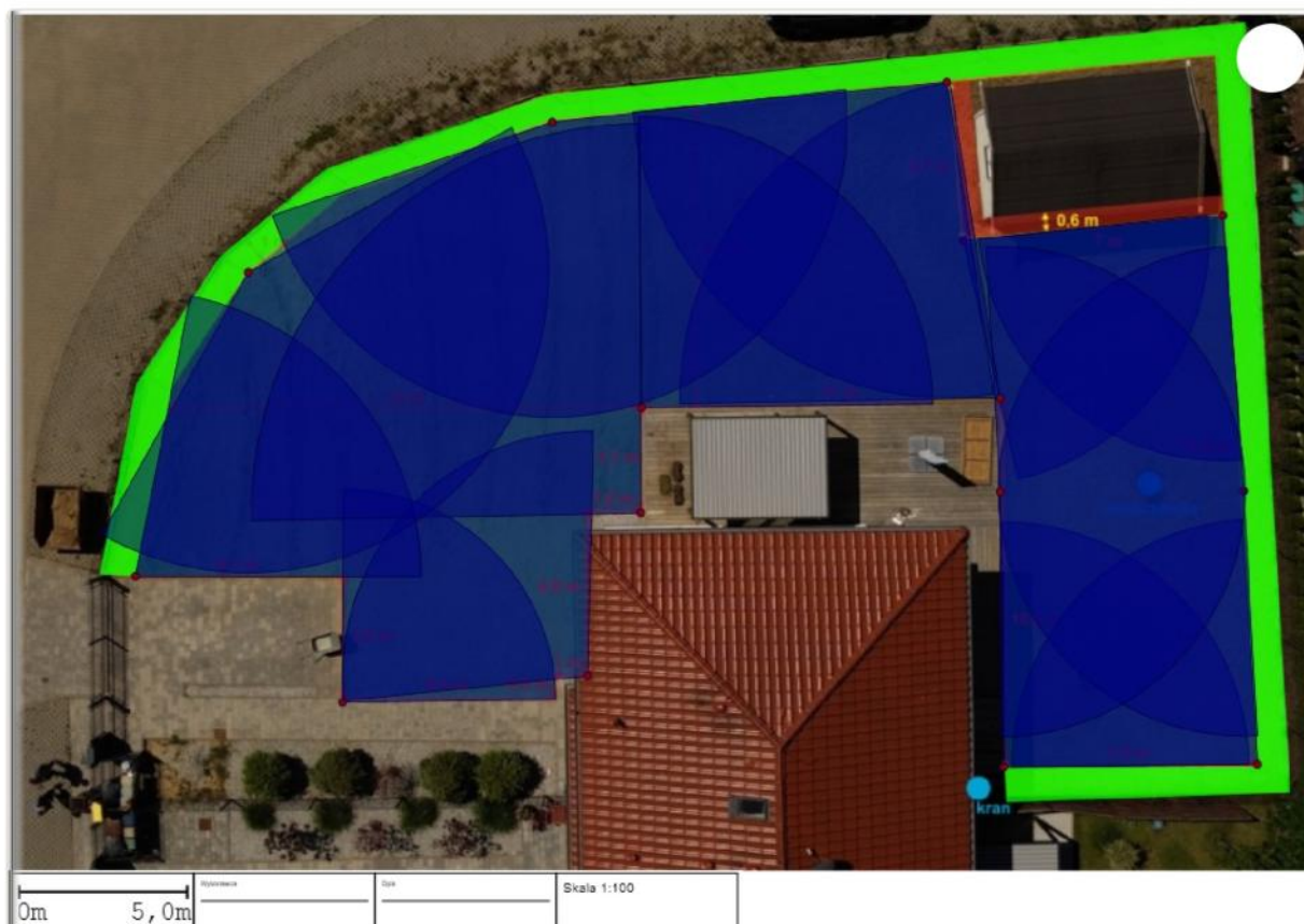
Rys. 1 — Projekt rozmieszczenia stref nawadniania na podkładzie ortofoto.
