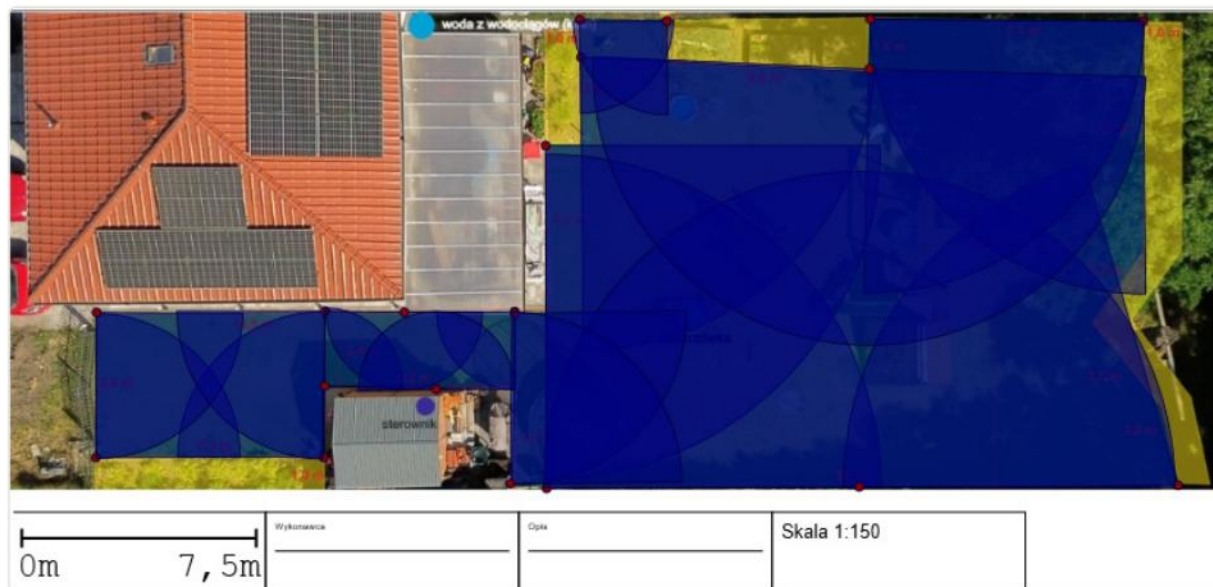
Rys. 1 — Projekt rozmieszczenia stref nawadniania na podkładzie ortofoto.
